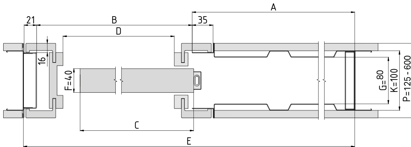
Horizontální řez pouzdra LATENTE STANDARD s dřevěným dveřním křídlem tloušťky 40 mm
