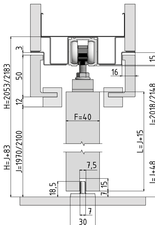
Vertikální řez pouzdra LATENTE STANDARD s dřevěným dveřním křídlem tloušťky 40 mm
